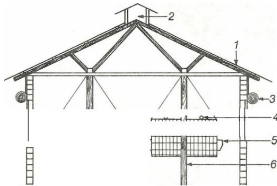
8. Figura 6.19.15. Detalles constructivos del galpón cerrado
