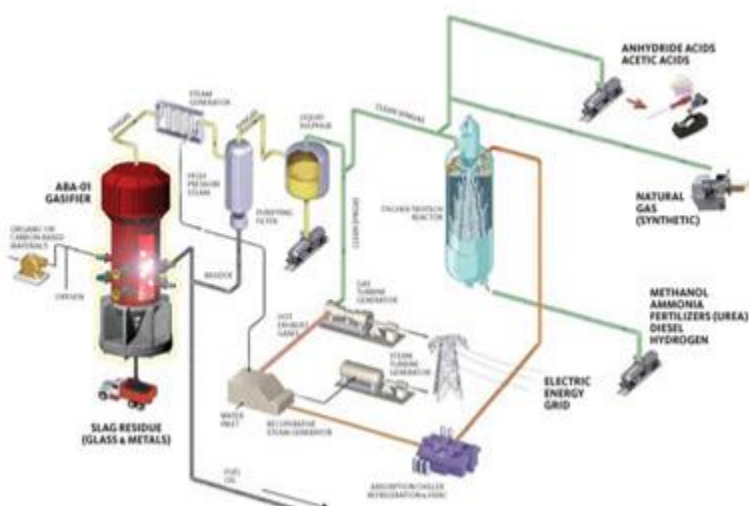
Figura 6.22.6. Esquemático de flujo usando Pirolisis
