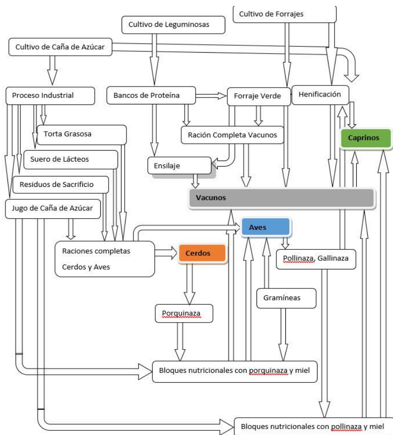
Figura 6.19.2. Diagrama de flujo de una Granja Integral Autosuficiente
