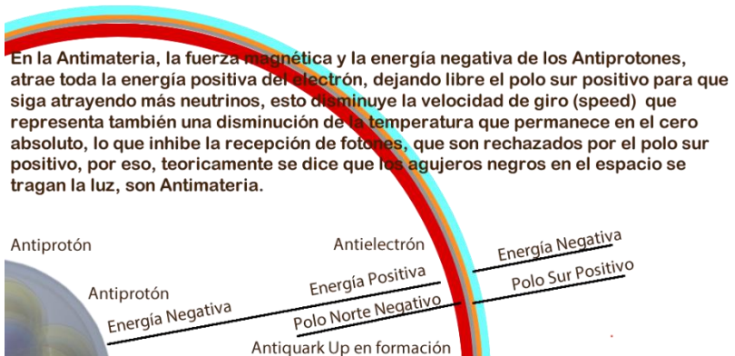
Figura 6.1.22. Comportamiento de la antimateria.
