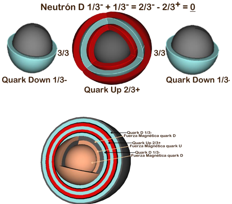
Figura 6.1.16. Neutrón completo
