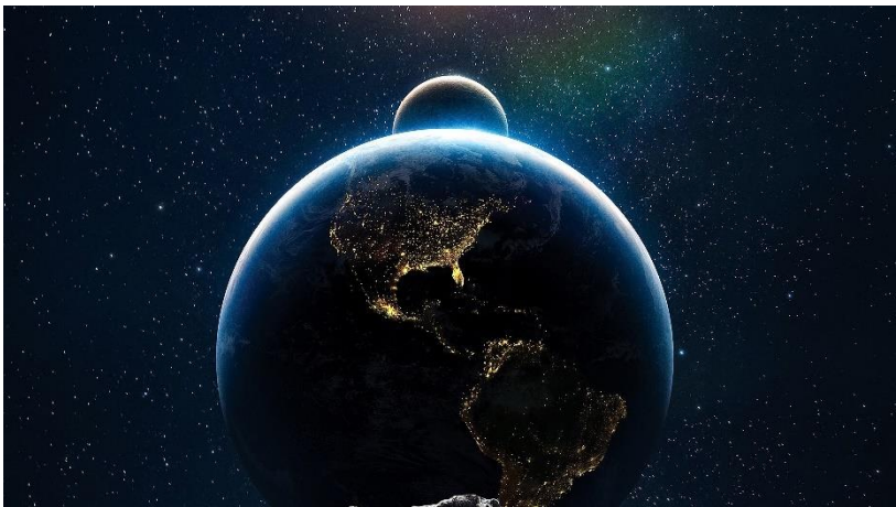
Figura 6.1.4. Planeta tierra y la luz
