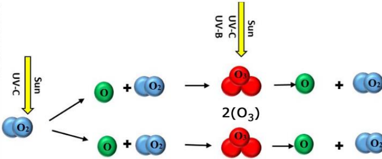
Figura 6.1.23. Oxígeno libera fotones y se convierte en ozono.
