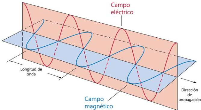
Figura 6.1.2. Descripción de una onda electromagnética
