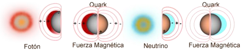
Figura 6.1.8. Descripción del fotón, el neutrino y la fuerza magnética que los sujeta
