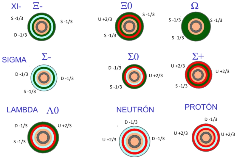
FIGURA 3.10.10. Los bariones
