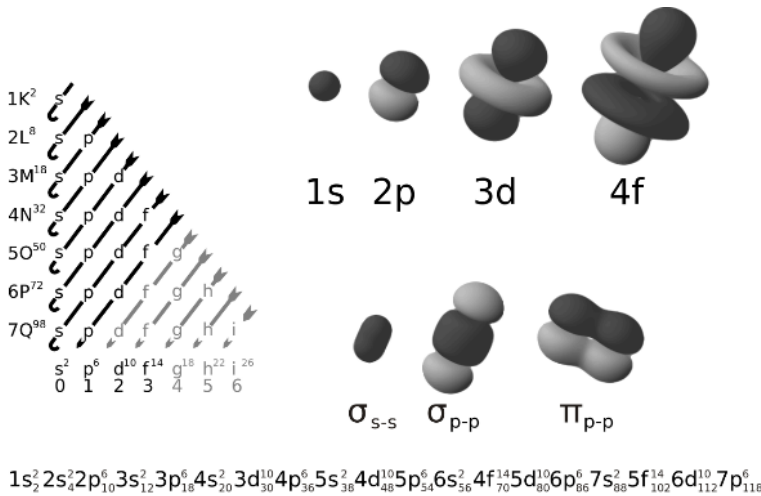
Figura 6.1.20. Orbitales en los átomos, definidos por el número de electrones.
