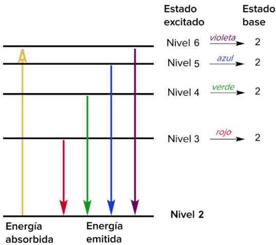
Figura 6.1.3. Espectroscopía, niveles de interacción de los fotones con átomos
