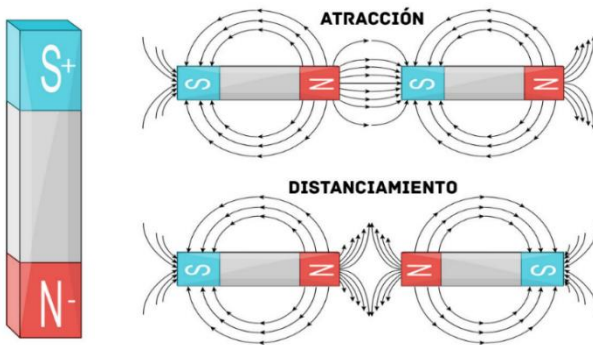
Figura 6.1.5. Ley del Magnetismo Universal
