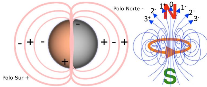
Figura 6.1.6. Descripción de la Fuerza Magnética
