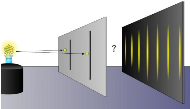
Figura 6.1.1. Descripción del fotón como onda y como partícula
