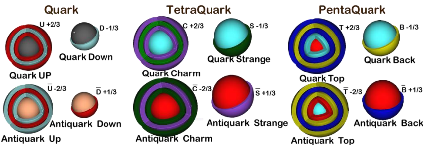
Figura 6.1.18. Diferentes tipos de quarks
