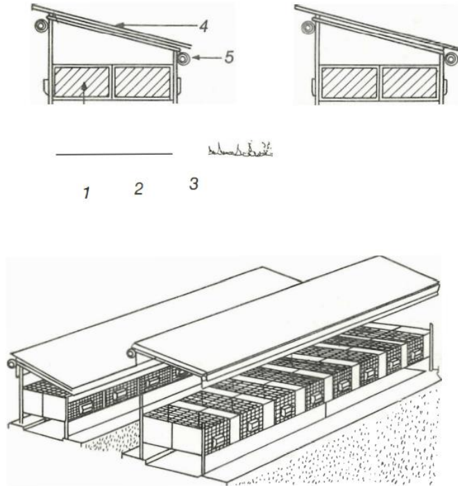
Figura 6.19.17. Vista lateral e isométrica de los galpones
