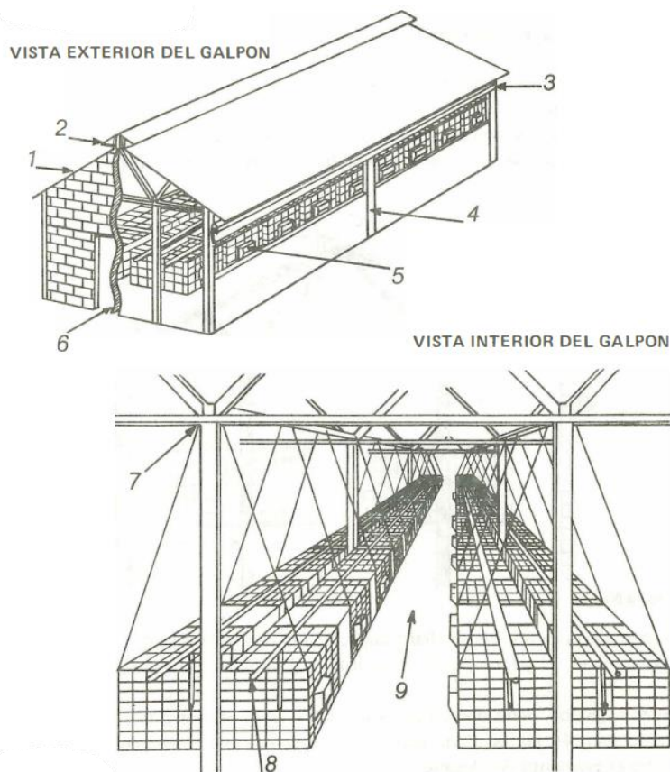
10. Figura 6.19.14. Detalles del Galpón Cerrado
