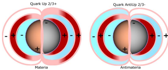
Figura 6.1.12. Descripción del Quark Up y el Anti-quark Up
