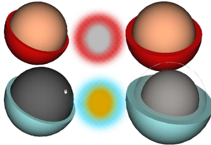
Figura 6.1.10. Aumento de energía en fotones y neutrinos
