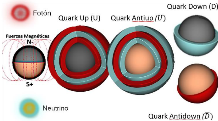
Figura 6.1.15. Descripción de la formación del quark up.
