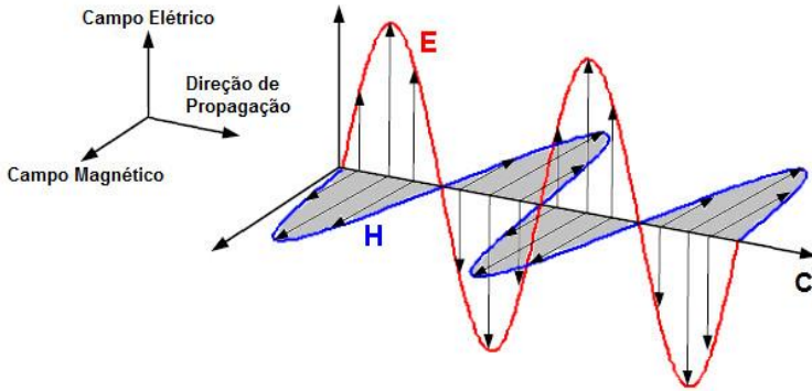
Figura 6.1.7. Descripción de una onda electromagnética
