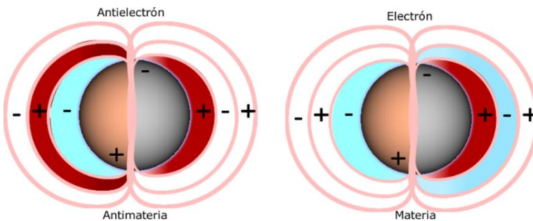
Figura 6.1.11. Electrón y Antielectrón
