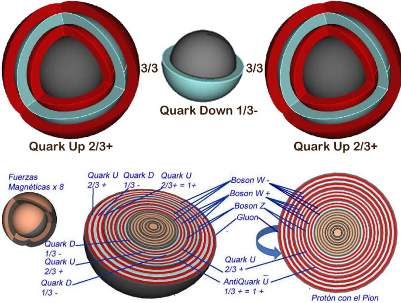
Figura 6.1.17. Neutrón, Pion, Protón y sus bosones
