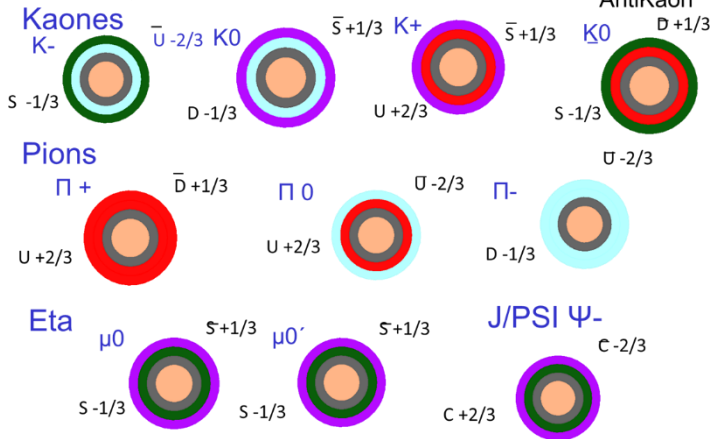
Figura 3.10.11. LOS Mesones
