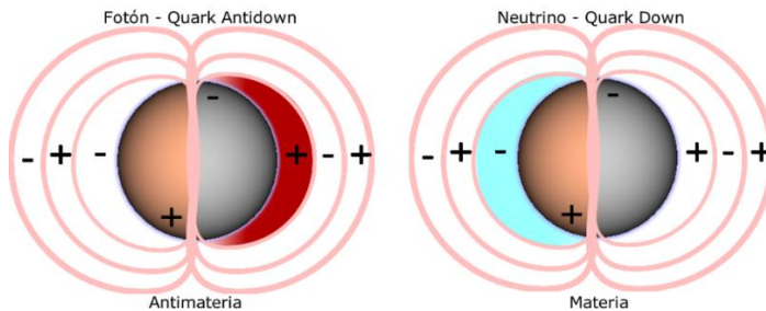
Figura 6.1.13. Descripción del Quark Up y el Anti-quark Up
