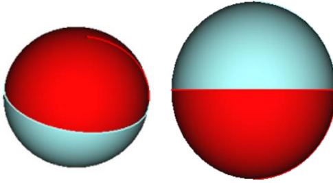
Figura 6.1.14. Tetraquarks y Pentaquarks
