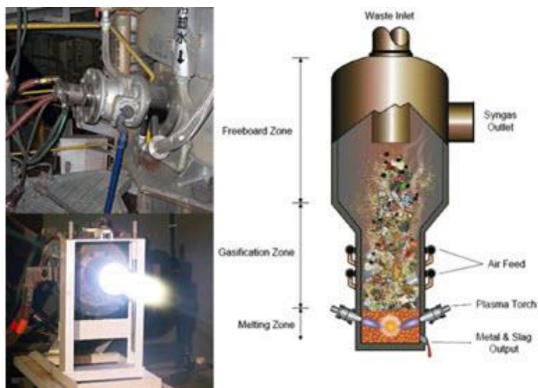
Figura 6.22.7. Esquemático del funcionamiento de la pirolisis con plasma
